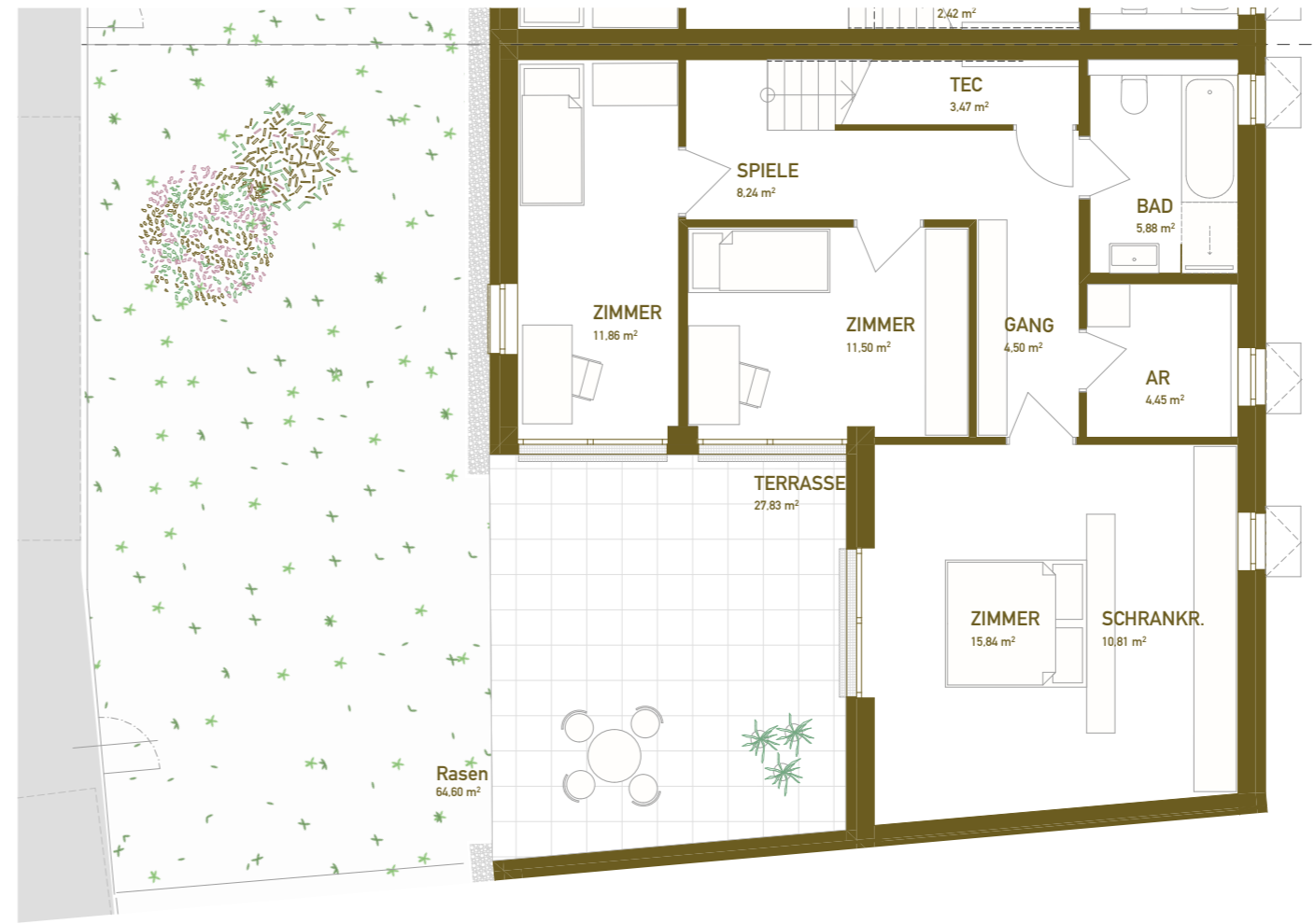
GRUNDRISS EBENE -01
